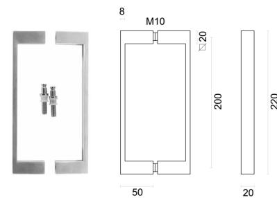
U-greep
