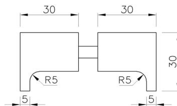
Deurknop
